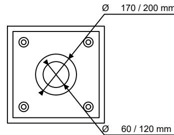
Placa metálica (Base)
