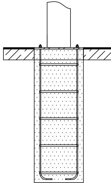
Det. Anclaje de Poste
