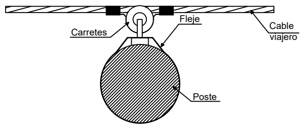
DET. 2 ESC: S/E
