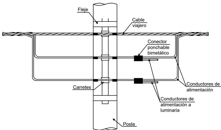
DET. 1 ESC: S/E
