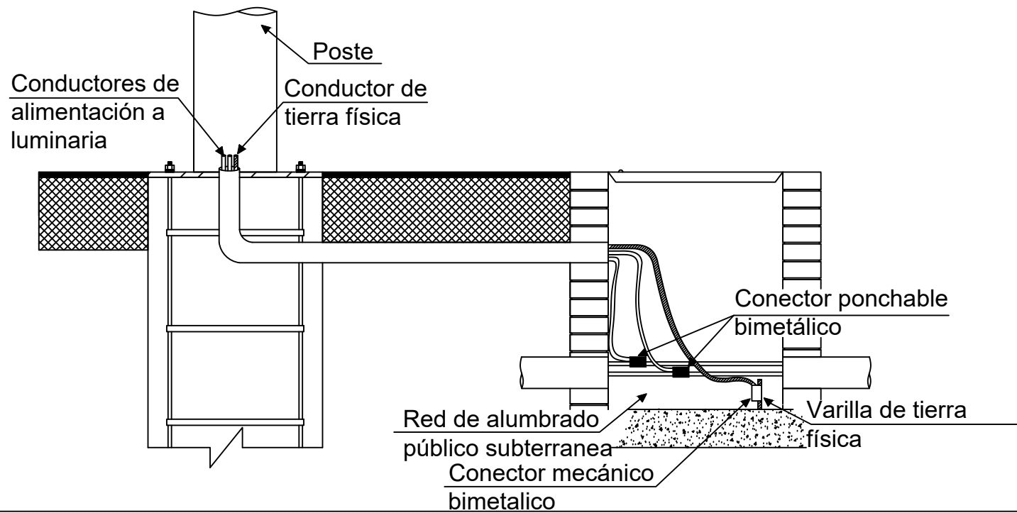
Detalle típico de alimentación subterránea con varilla de tierra física
