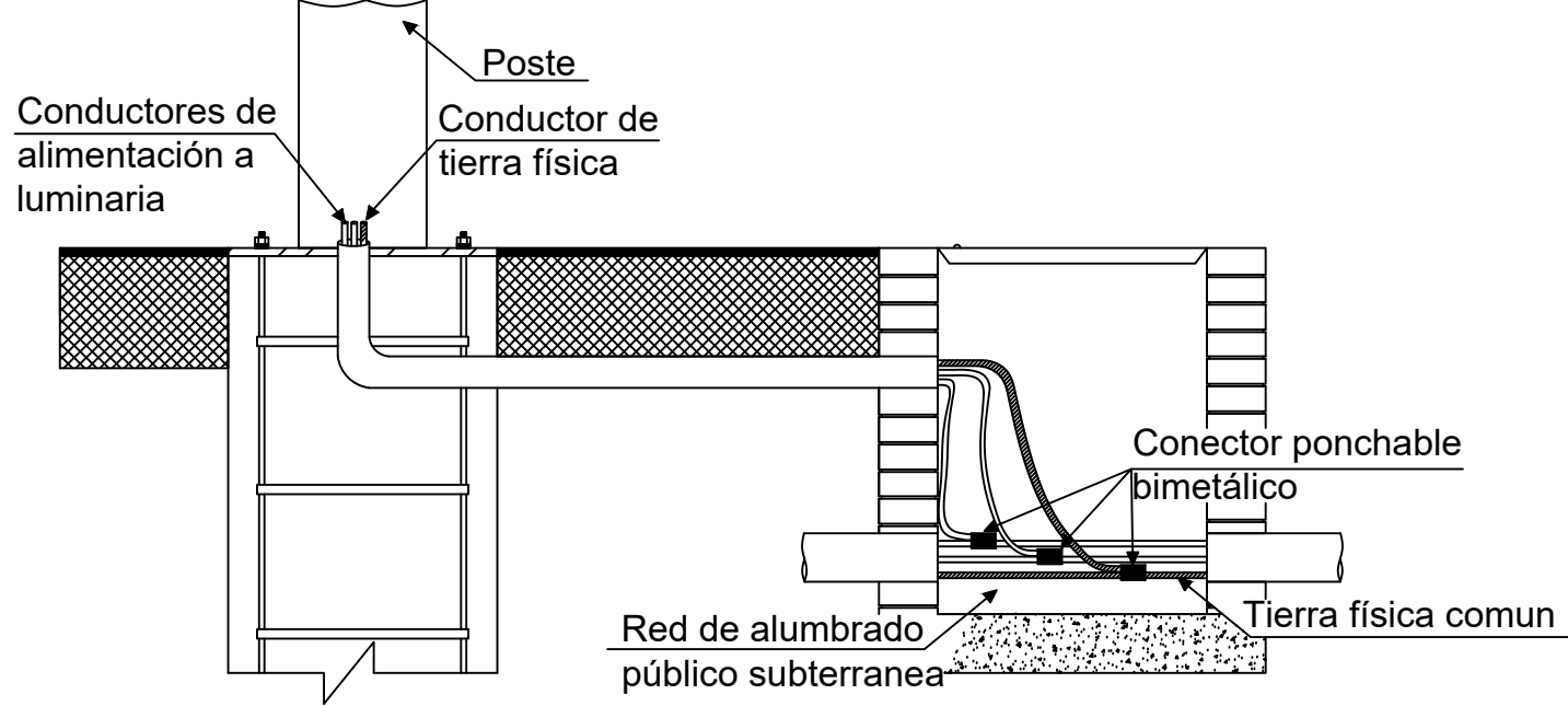
Detalle típico de alimentación subterránea con tierra común
