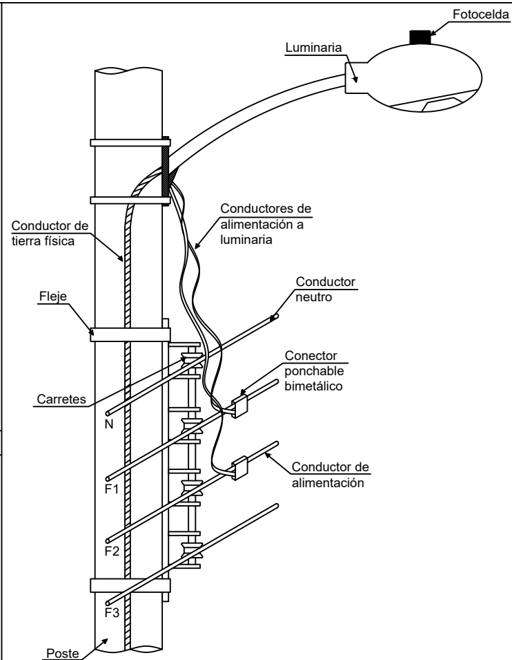
DET. 3 Vista lateral
