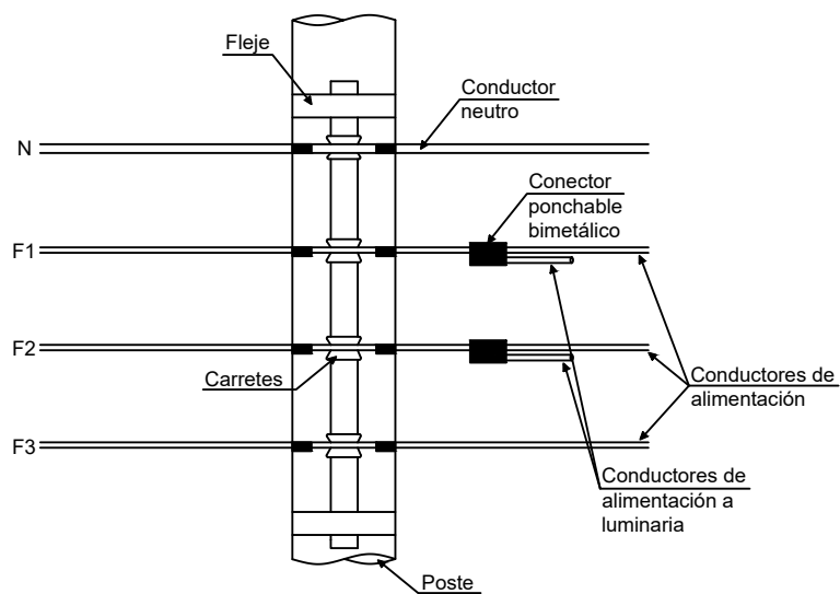
DET. 1 Vista frontal de instalación a red eléctrica
