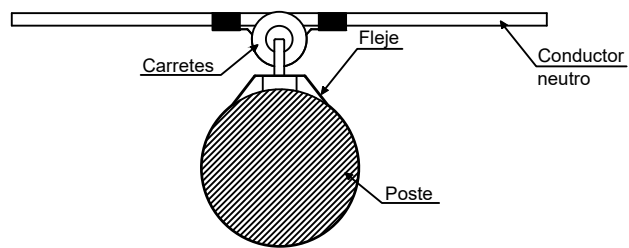
DET. 2 Vista superior de instalación a red eléctrica
