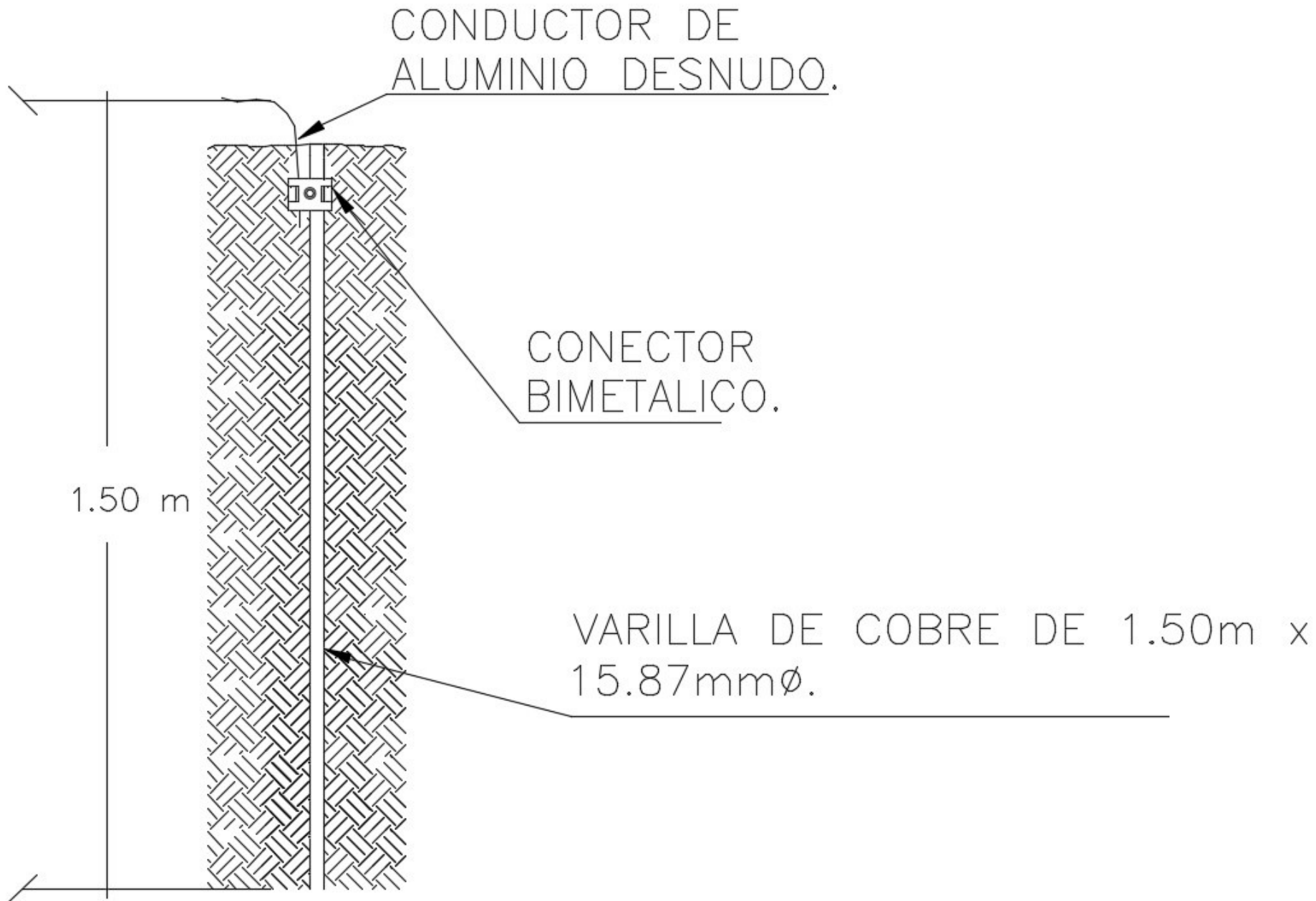
DETALLE DE VARILLA DE SISTEMA DE TIERRAS
